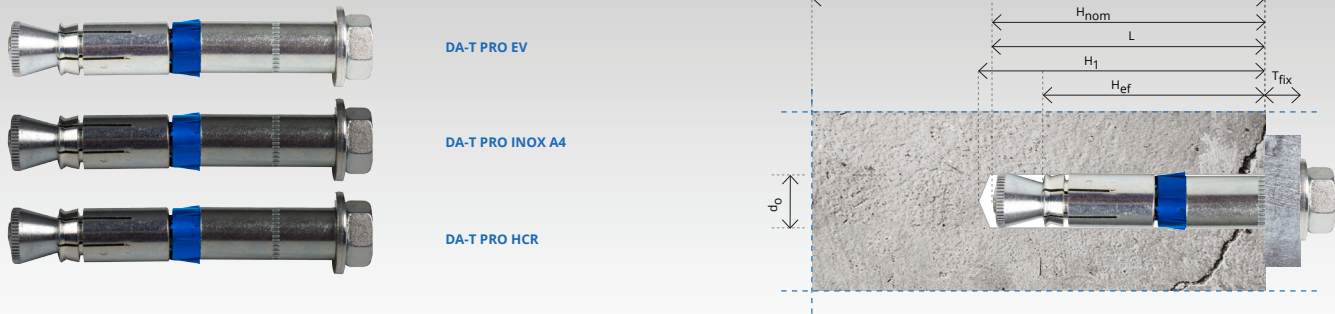
DA-T PRO ACHTERINSNIJDEND ANKER EV
